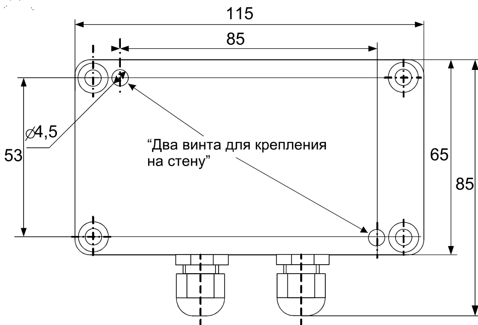
Рисунок 5.1 – Схема крепления
